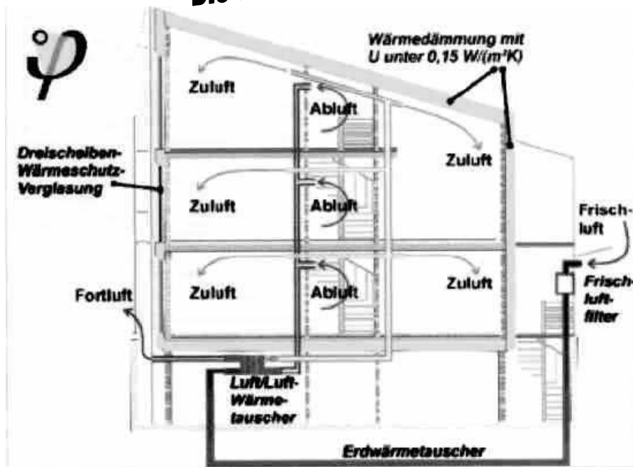
Das Prinzip eines Passivhauses
